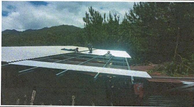
Foto 1: el estado de la laminas esta en mal estado por tal razon es necesario el cambio de laminas por nuevas y tambien el cambio de la estructura metalicas para darle un mejor aspecto al corredor de la escuela.
