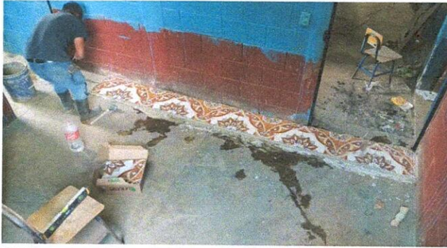
Foto7: inicio de colocacion de piso ceramico en la cocina
